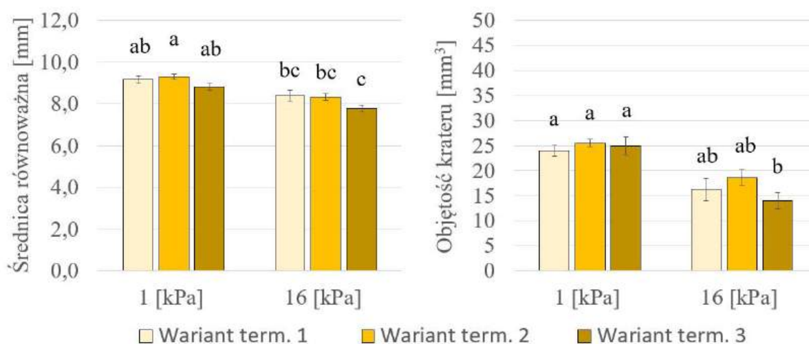
Rys. 9. Średnica równoważna i objętość kraterów formowanych na piasku gliniastym przy wilgotności odpowiadającej potencjałowi wody glebowej równemu 1 kPa oraz 16 kPa (za pomocą wąsów przedstawiono błąd standardowy, SE). Litery umieszczone na rysunku odpowiadają wynikom testu post-hoc Tukeya ( p < 0,05 ) przeprowadzonego na komplecie danych, wskazując istotne statystycznie różnice między poszczególnymi wariantami eksperymentu.
