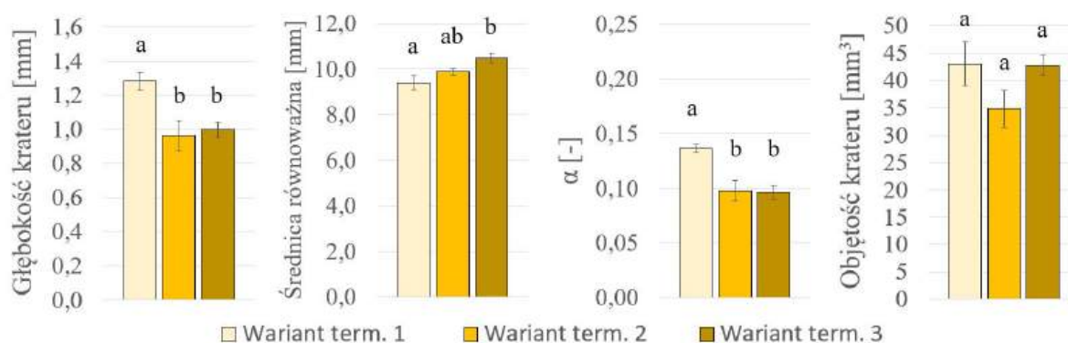
Rys. 8. Wielkości charakteryzujące kratery formowane na pyłe gliniastym przy wilgotności odpowiadającej potencjałowi wody glebowej równemu 1 kPa (za pomocą wąsów przedstawiono błąd standardowy, SE). Litery umieszczone na rysunku odpowiadają wynikom testu post-hoc Tukeya ( p < 0,05 ) przeprowadzonego na komplecie danych, wskazując istotne statystycznie różnice między poszczególnymi wariantami eksperymentu.
