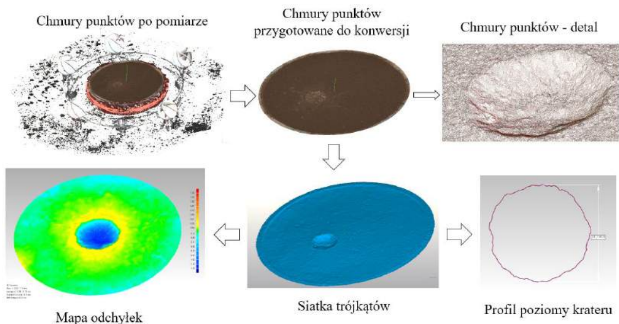
Rys. 7. Sekwencja analizy obrazów kraterów uzyskanych przy pomocy skanera powierzchni (Foto: zdjęcie własne).
