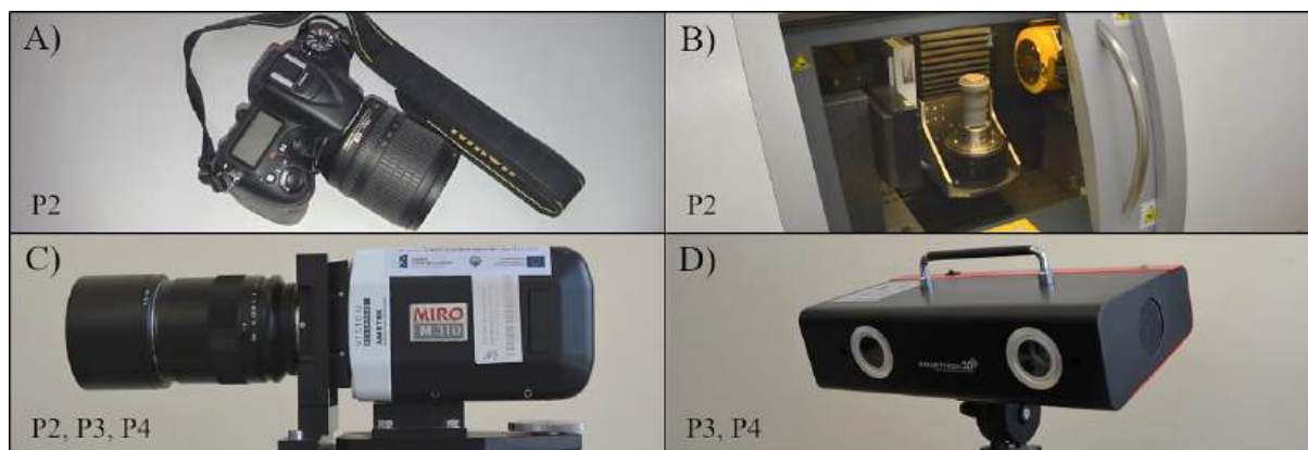
Rys. 6. Zestawienie aparatury pomiarowej wykorzystanej w badaniach: A) aparat cyfrowy Nikon D7100 ( P2 ), B) mikrotomograf GE Nanotom 180S ( P2 ), C) szybka kamera Phantom Miro 310 ( P2, P3, P4 ), D) skaner powierzchni Scan3D UNIVERSE 10 Mpix ( P3, P4 ) (Foto: zdjęcia własne).
