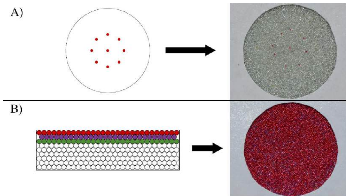
Rys. 4. Przykłady złóż modelowych przygotowanych ze szklanych kulek: A) schemat koncentrycznego wzoru z markerów na powierzchni złoża prostego oraz zdjęcie złoża przed uderzeniem kropli, B) schemat prezentujący koncepcyjny układ monowarstw na powierzchni złoża oraz zdjęcie złoża przed uderzeniem kropli (Foto: zdjęcia własne).
